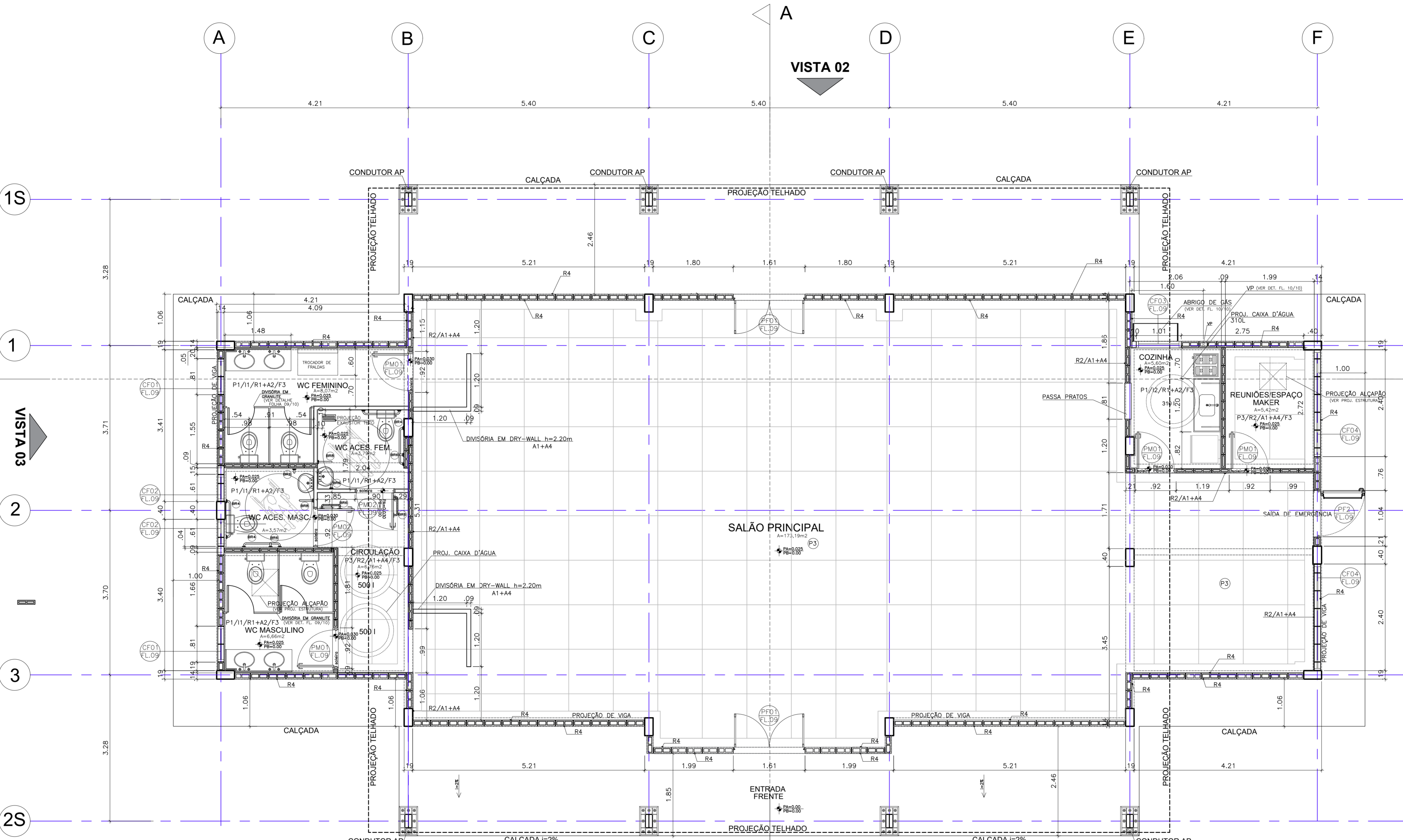
PLANTA ESC.: 1:50
