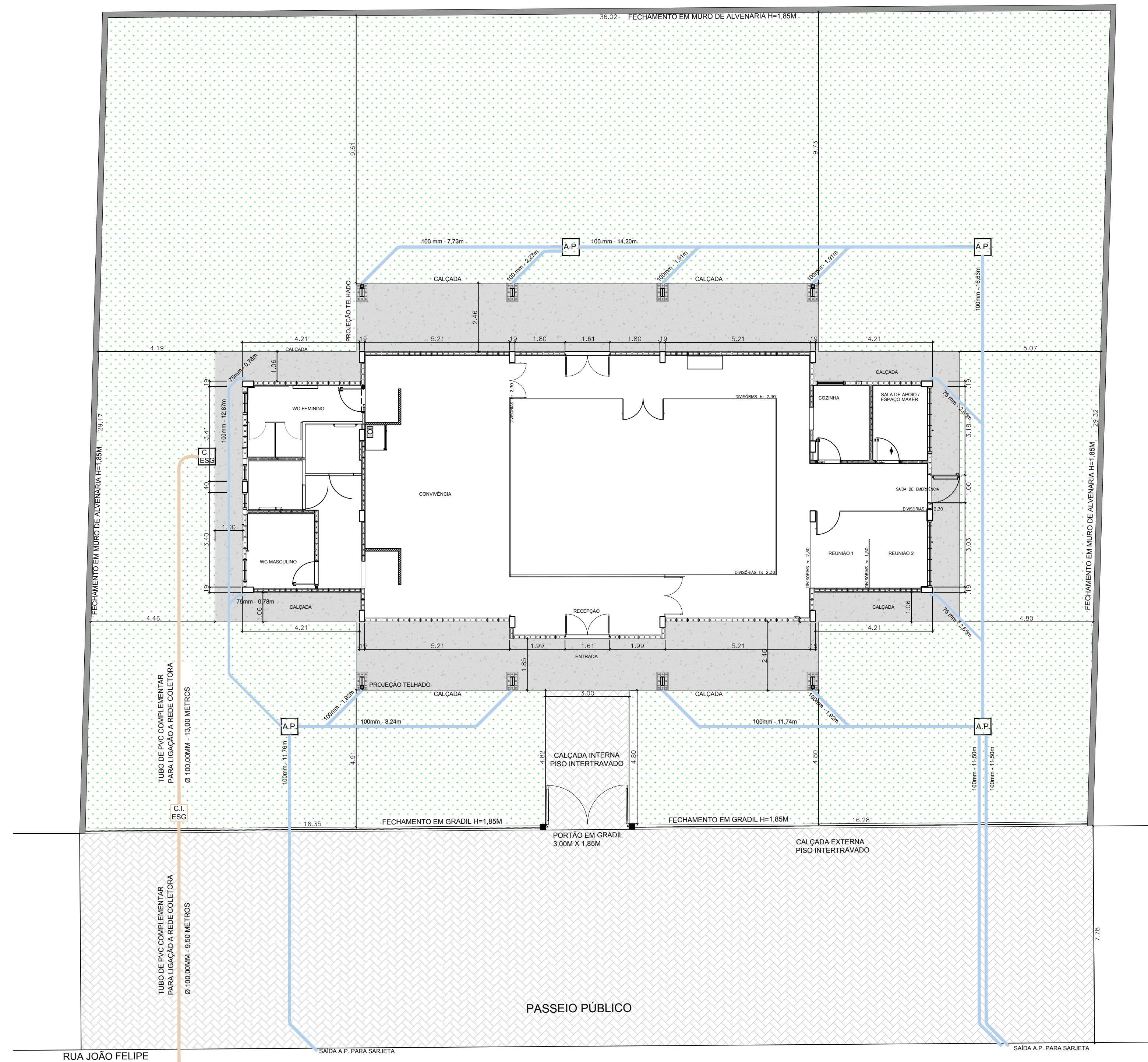
IMPLANTAÇÃO DA CONSTRUÇÃO ESCALA: 1:100
