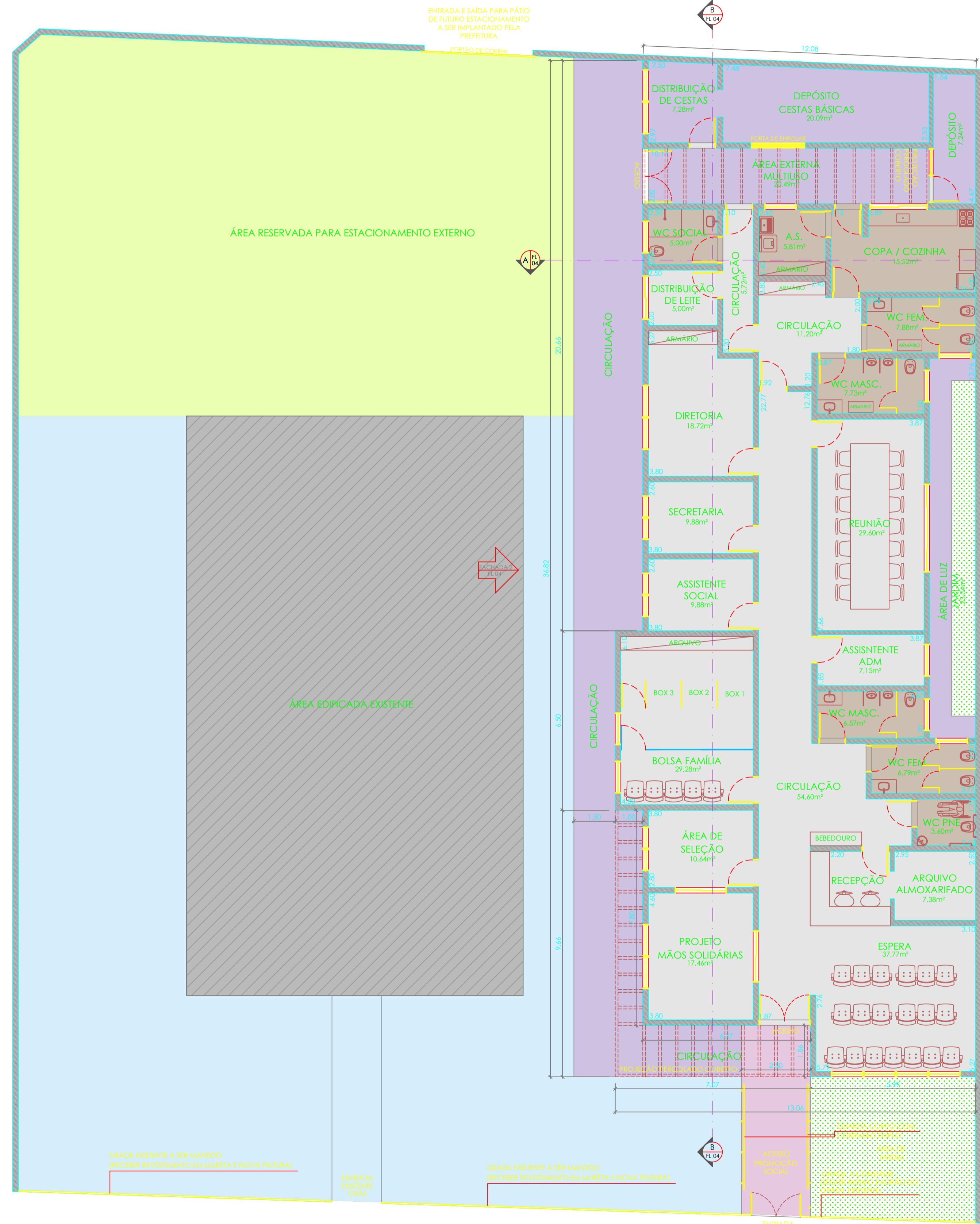
PLANTA BAIXA ESC 1:100
