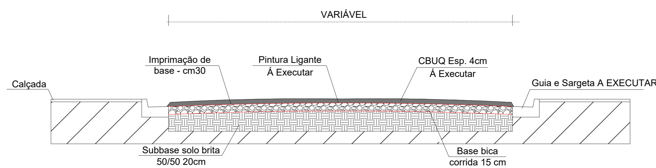
CORTE S/ ESCALA
