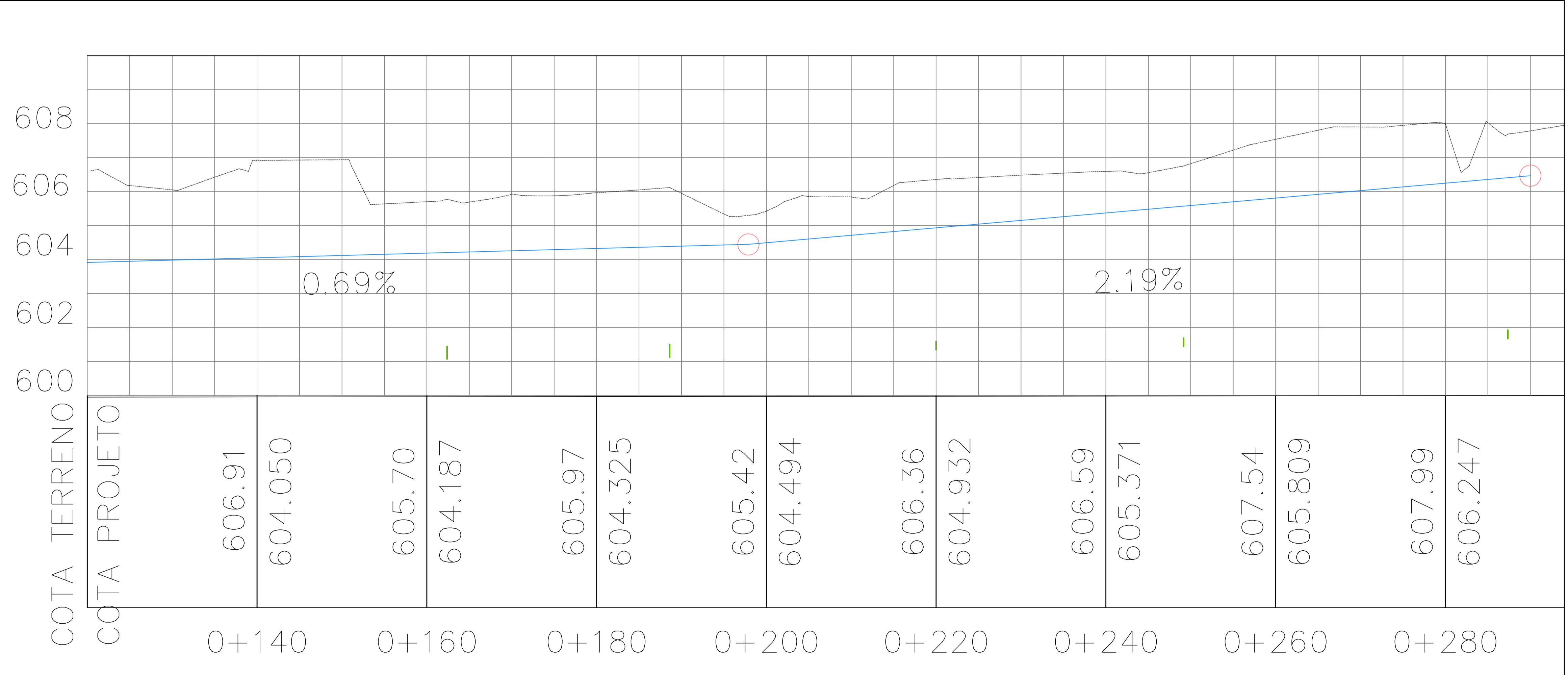
PERFIL (DEFORMAÇÃO VERTICAL = 2x) ESC 1:200
