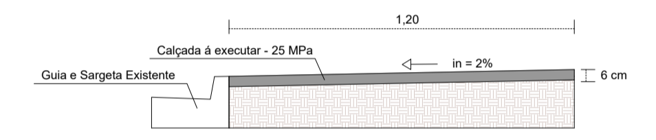
DETALHE CALÇADA - S/ ESCALA
