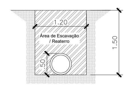
DETALHE DE ESCAVAÇÃO DE VALA S/ ESCALA Área de escavação: 1,80 m² Área de reaterro: 1,80 m²
