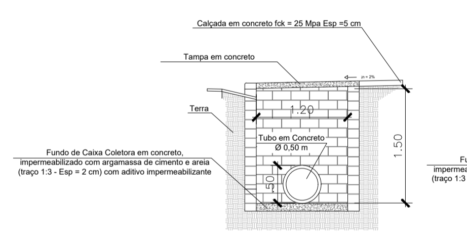
DETALHE DE CAIXA COLETORA (BOCA DE LOBO) S/ ESCALA
