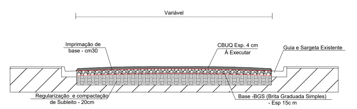
DETALHE DE PAVIMENTAÇÃO S/ ESCALA
