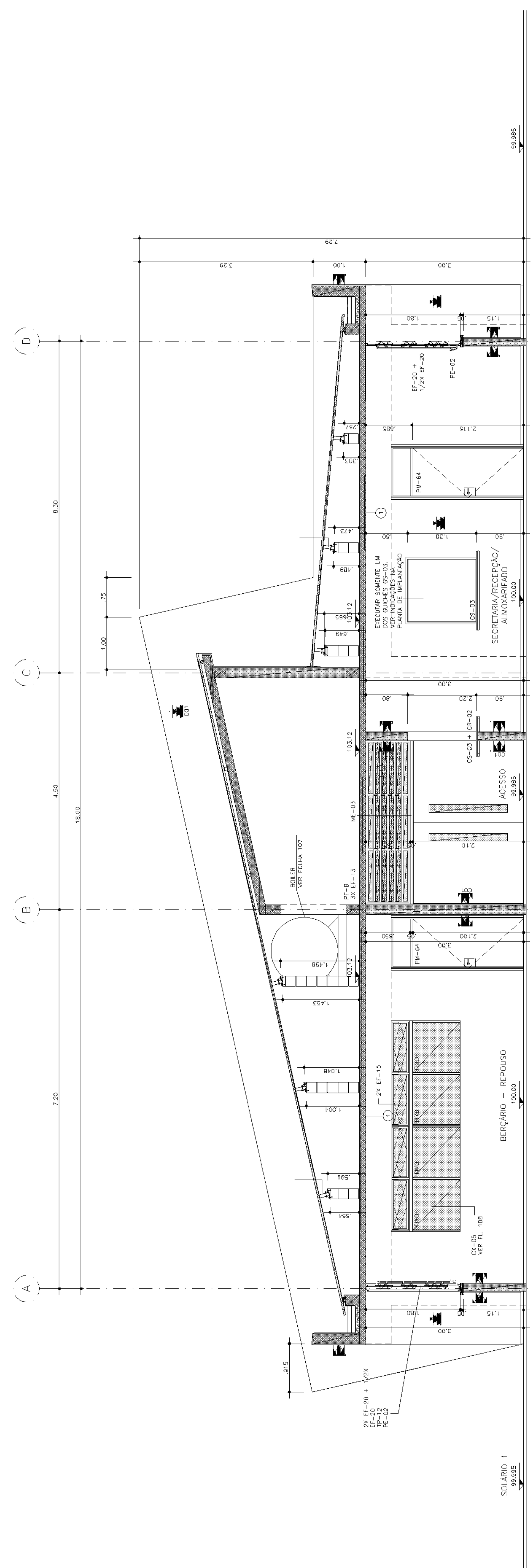
CORTE A
