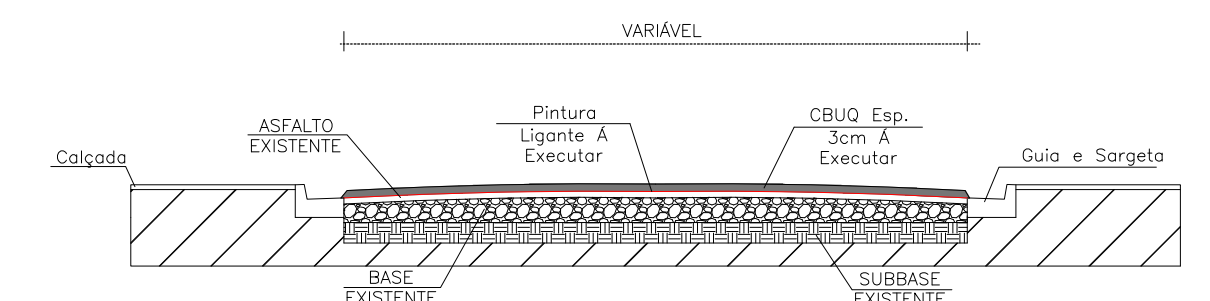
CORTE S/ ESCALA
