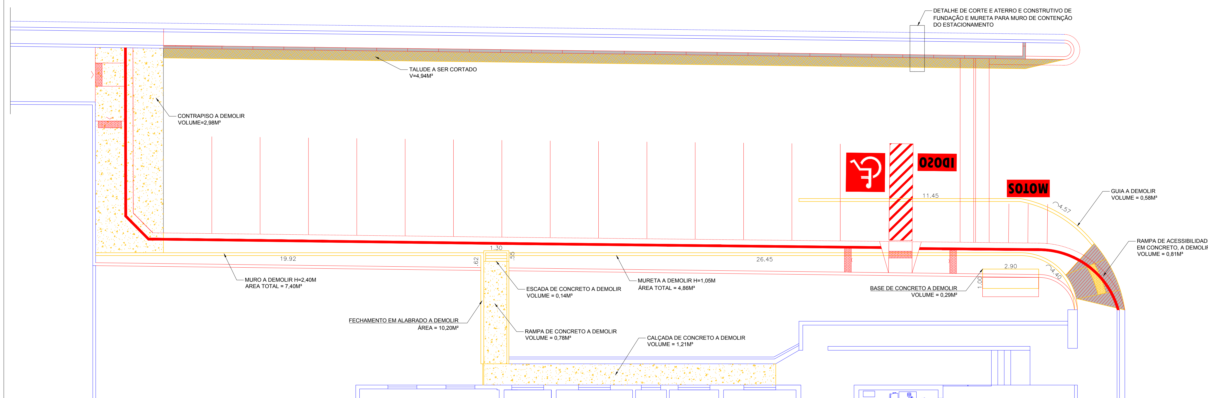
DETALHE DE ATERRO PARA E CONSTRUÇÃO DA MURETA DE CONTENÇÃO/GUARDA-CORPO DA CALÇADA
