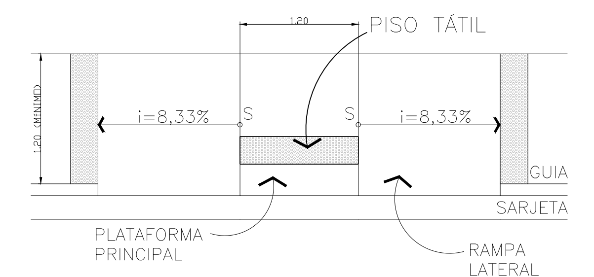
DETALHE RAMPAS PNE SEM ESCALA
