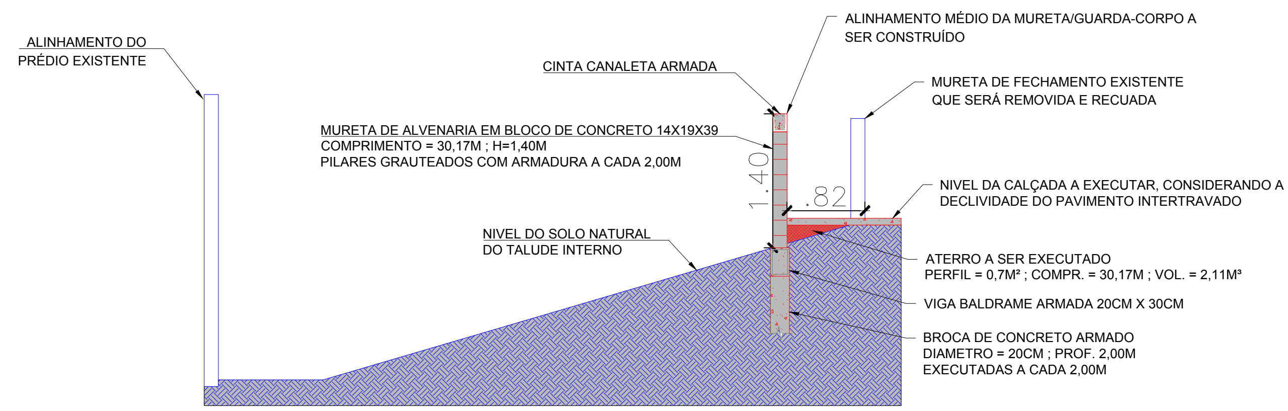
DETALHE DE ATERRO PARA E CONSTRUÇÃO DA MURETA DE CONTENÇÃO/GUARDA-CORPO DA CALÇADA
