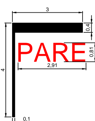
DETALHE - SINALIZAÇÃO HORIZONTAL "PARE"
