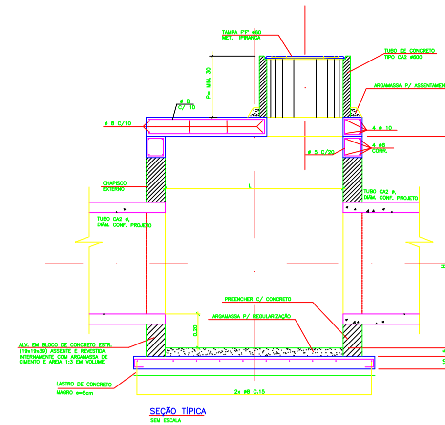
SEÇÃO TÍPICA SEM ESCALA
