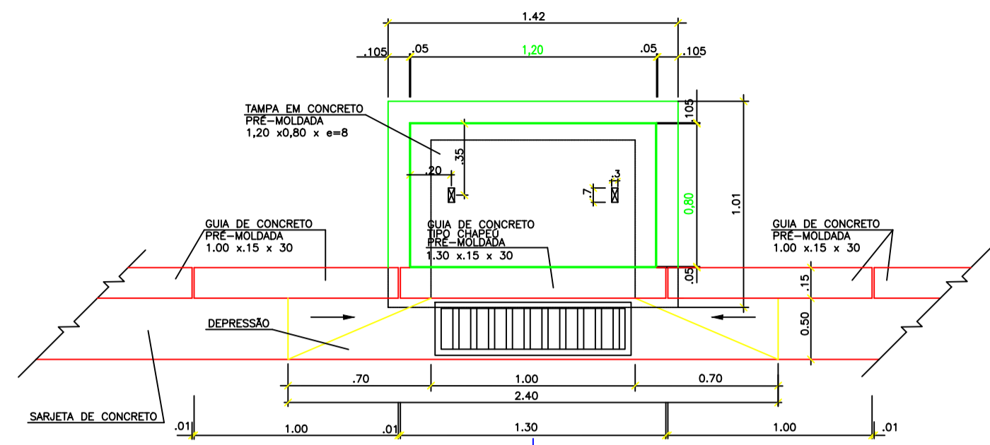
PLANTA - COTA SUPERIOR SEM ESCALA DETALHAMENTO DA BOCA DE LOBO
