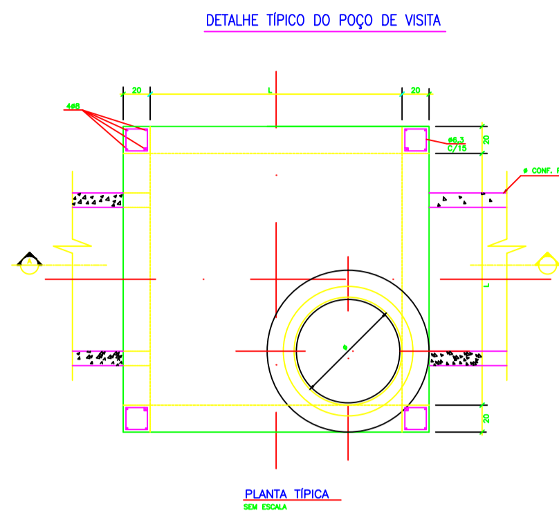
PLANTA TÍPICA SEM ESCALA
