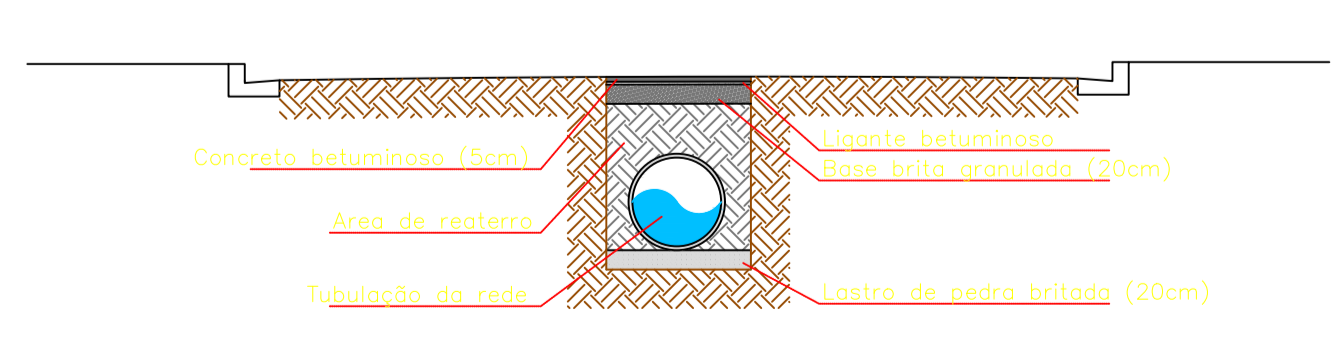
DETALHES DO PERFIL TRANSVERSAL DA REDE SEM ESCALA
