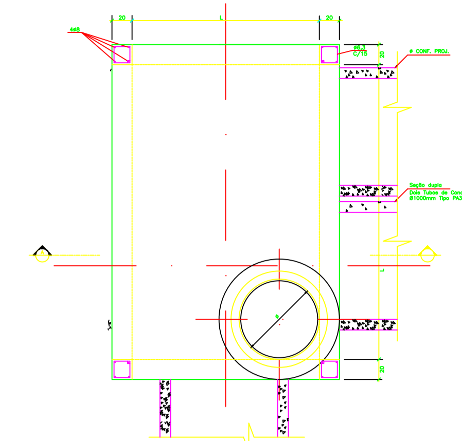
DETALHE 1 - POÇO DE VISITA 6 SEM ESCALA
