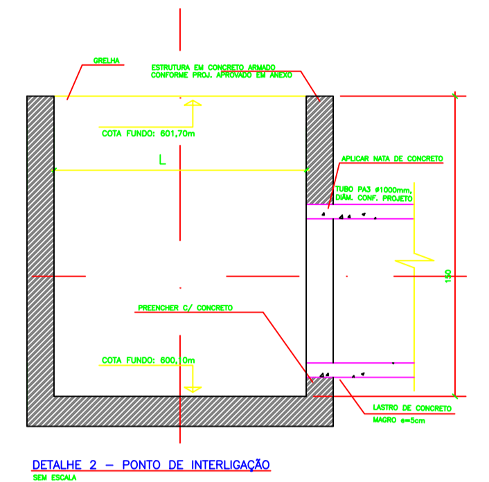
DETALHE 2 - PONTO DE INTERLIGAÇÃO SEM ESCALA
