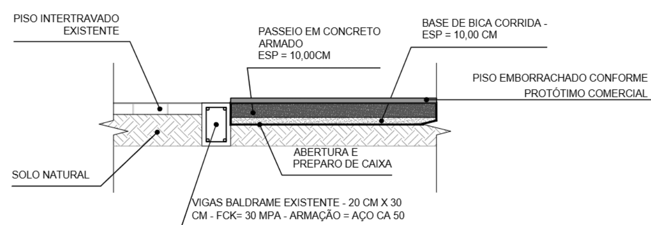
DETALHE PARA EXECUÇÃO DE PISO DE CONCRETO S/ ESCALA
