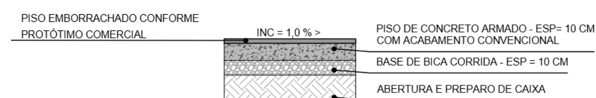
DETALHE DE EXECUÇÃO DE PISO DE CONCRETO ARMADO S/ ESCALA
